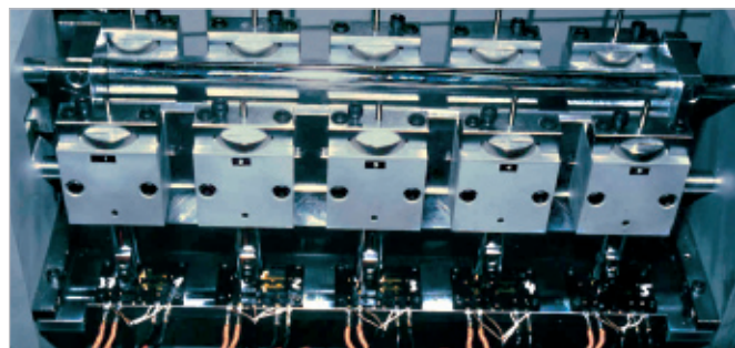
Schwing-Reib-Verschleiß-Prüfstand
