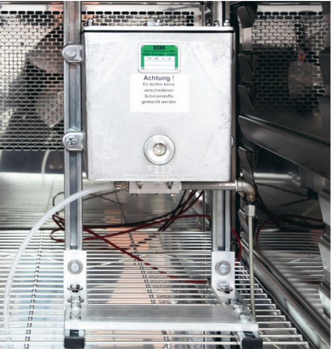
轮缘润滑测试台
